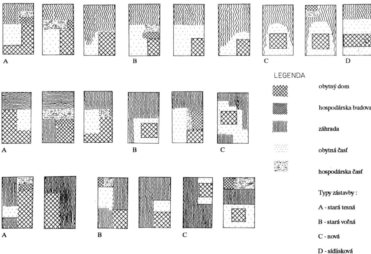
Najvhodnejšie pôdorysy zástavby: 1. na rovine, 2. v pahorkatine, 3. vo vrchovine
